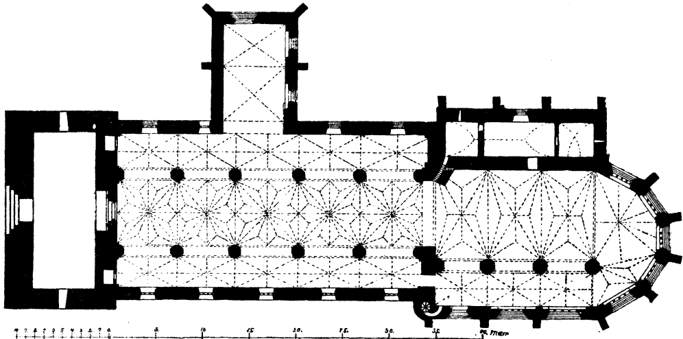
Fig. 1. Grundriß der Pfarrkirche St. Marien zu Angermünde.
